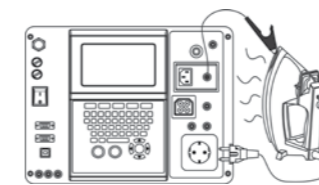
Berührungsableitstromprüfung für Geräte der Klasse II
