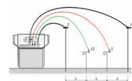
Messung des spezifischen Erdwiderstands
