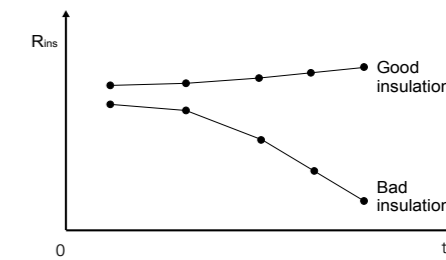
Typische Ergebnisse bei der Stufenspannungsmessung
