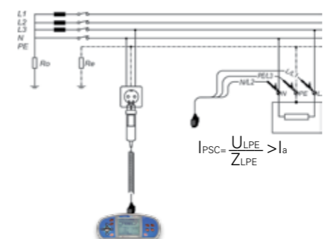
Schaltung für die Messung der Fehlerschleifenimpedanz
