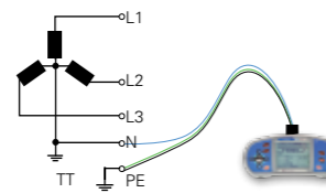
Zweileitermethode (Prüfung zwischen N und PE)
