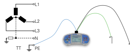
Dreileitermethode (Prüfleiter an Hilfsleiter in Dreieck-Schaltung)
