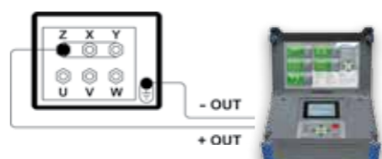
Messung des Isolationswiderstands von Induktionsmotoren zwischen allen drei Phasen gegenüber dem Metallgehäuse
