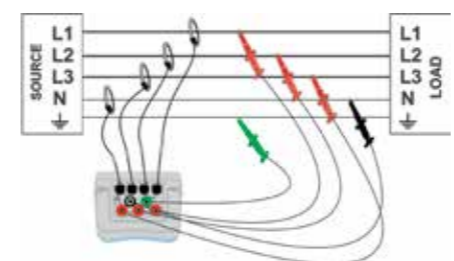
Anschluss an ein dreiphasiges 4-Leitersystem
